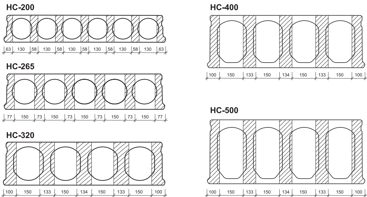
Rys. 17. Maksymalna wielkość otworów wykonywanych w osi kanałów płyty
