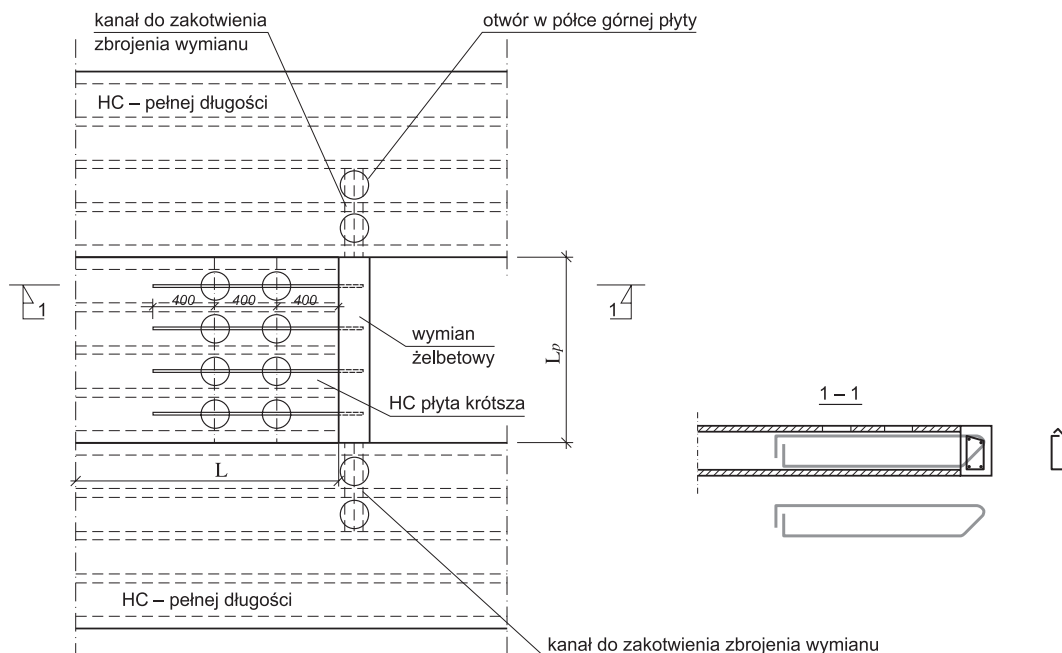
Rys. 25. Konstrukcja otworu w stropie z zastosowaniem wymianu żelbetowego
