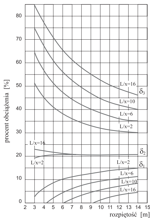
Rys. 30. Współczynnik rozdziálu obciążenia punktowego
