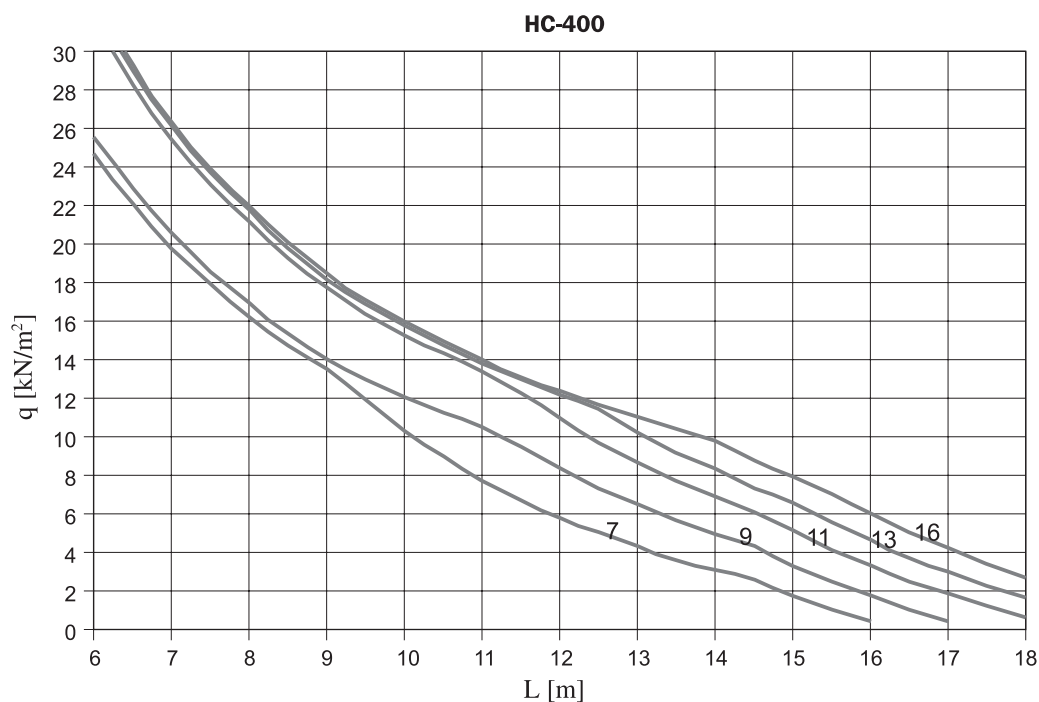
Rys. 13. Dopuszczalne, charakterystyczne obciążenia zewnętrzne p_k [kN/m²] płyt HC-400.
