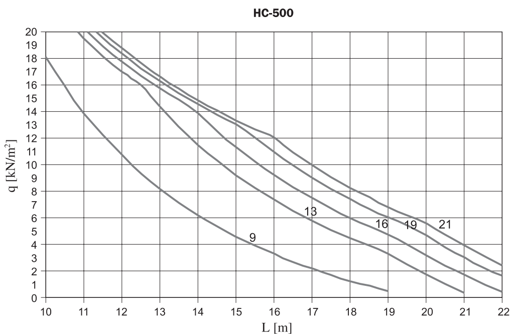
Rys. 15. Dopuszczalne, charakterystyczne obciążenia zewnętrzne q [kN/m 2 ] płyt HC-500.
