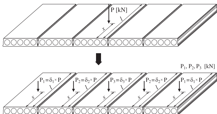
Rys. 29. Rozdział obciążenia punktowego na płyty sąsiadujące
