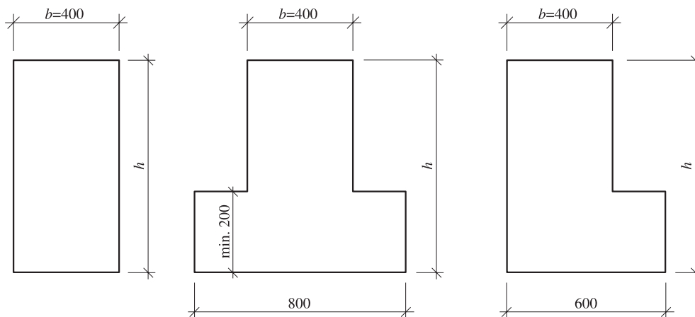
Rys. 5. Belki o szerokości b = 400 mm
