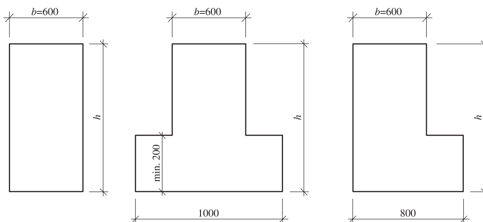
Rys. 7. Belki o szerokości b = 600 mm
