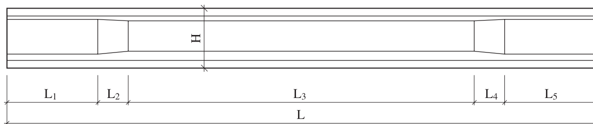
Rys. 3. Dźwigar o pasach równoległych – wersja z blokami podporowymi
