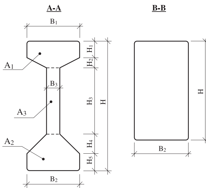
Rys. 2. Widok i przekroje dźwigara SI
